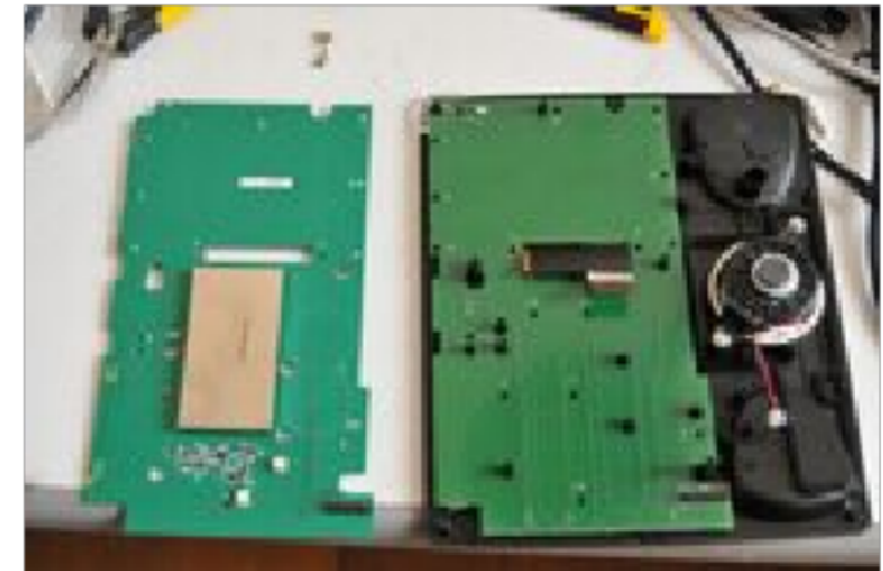
À gauche : version modifiée du plus grand circuit imprimé du téléphone (avec dispositif de surveillance) sans la batterie. À droite : version non modifiée.
