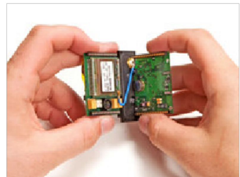
Module d'émission-réception (ouvert)
