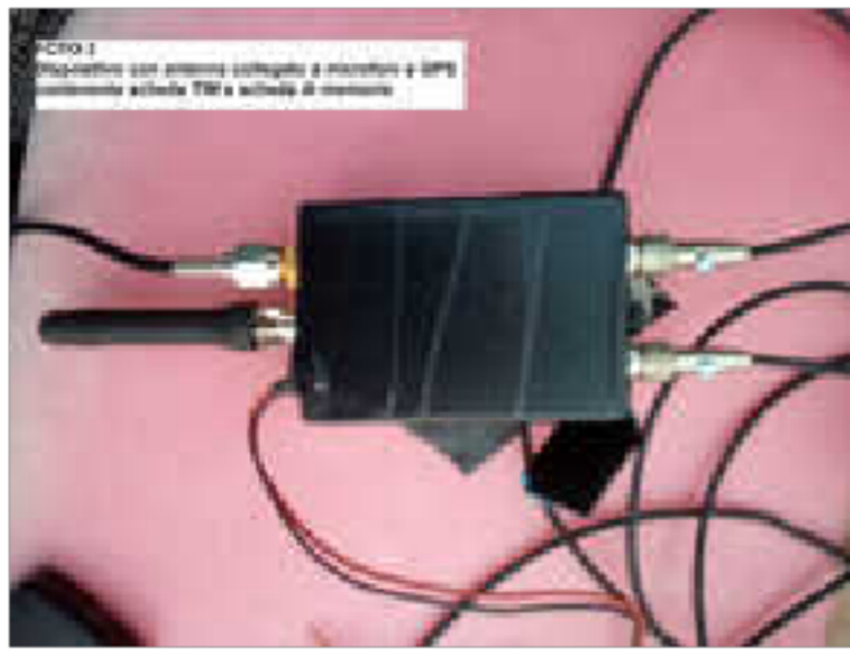
le dispositif avec antenne relié à micros et GPS. Il contenait aussi une SIM et une carte mémoire.
