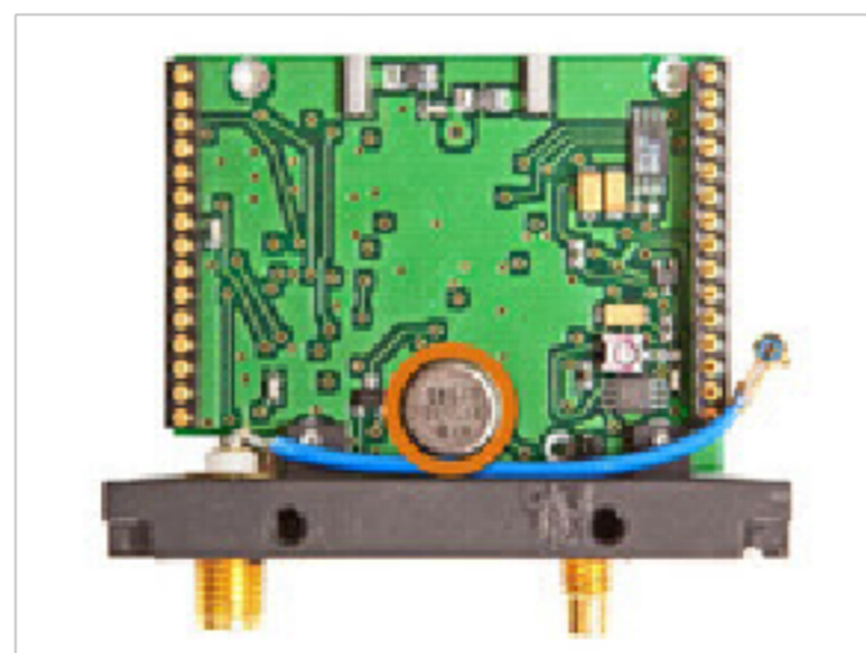
Module permettant la transmission par ondes radio (autre côté)
