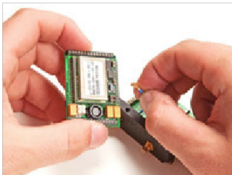
Module d'émission-réception (ouvert)
